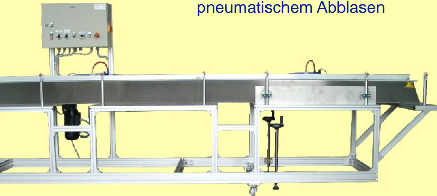
Bandablagetisch mit Links-Rechtslauf des Transportbandes
