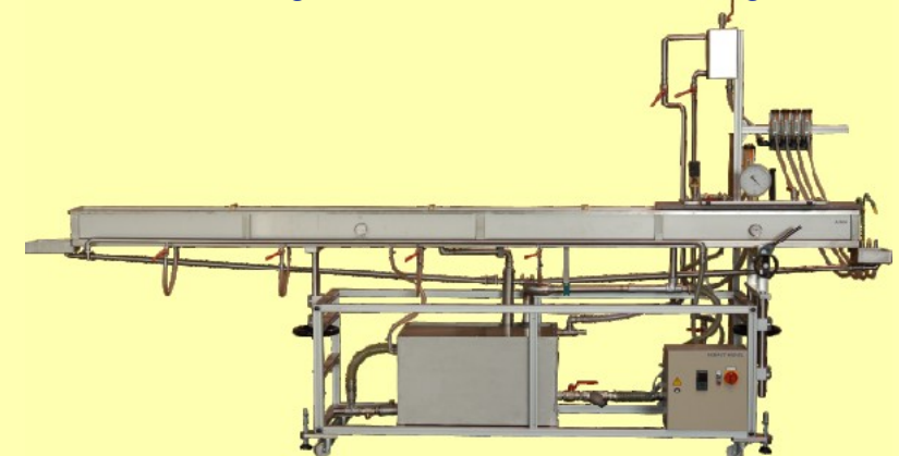
Vakuumtank mit elektronischer Vakuumregelung
